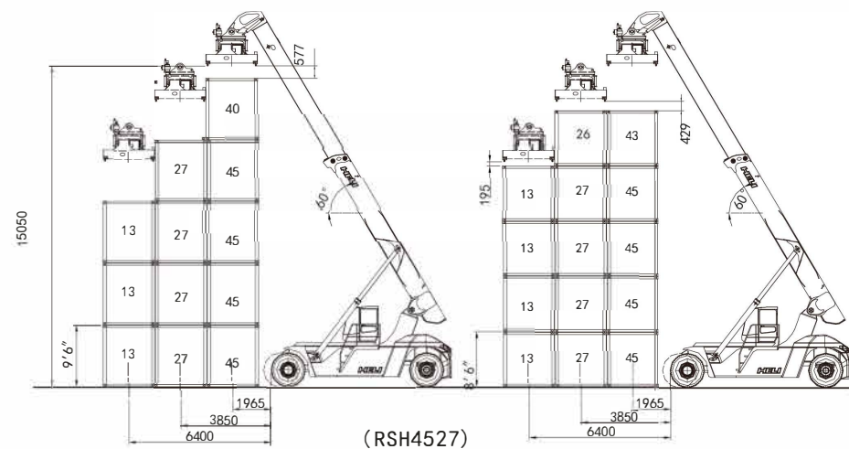
载荷图 Load diagram
